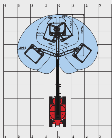
Option 3D: Drehung des Korbarms
